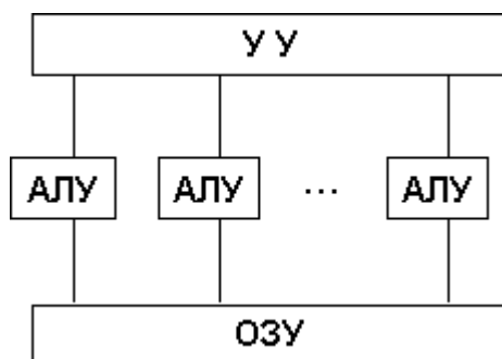
Рис. 3. Архитектура с параллельным процессором
