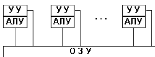
Рис. 2. Архитектура многопроцессорного компьютера
